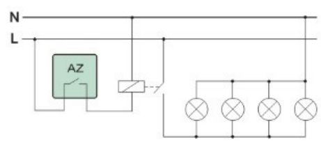
Układ sterowania stycznikiem załączającym odbiorniki o łącznym poborze prądu przewyższającym dopuszczalne obciążenie styku automatu zmierzchowego
